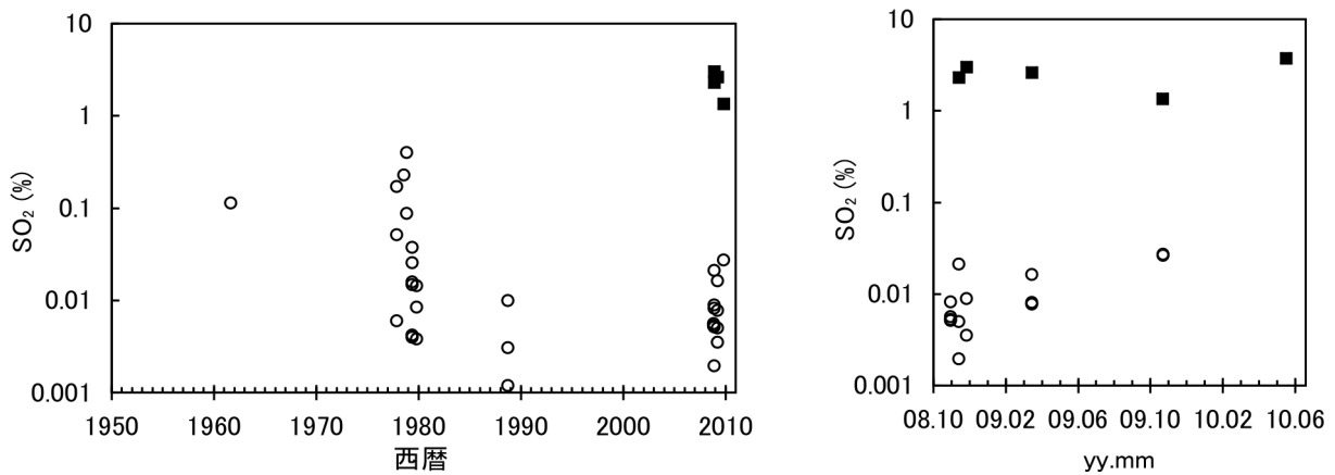
図 2 火山ガス中 \text{SO}_2 濃度 (黒四角は新噴気)
