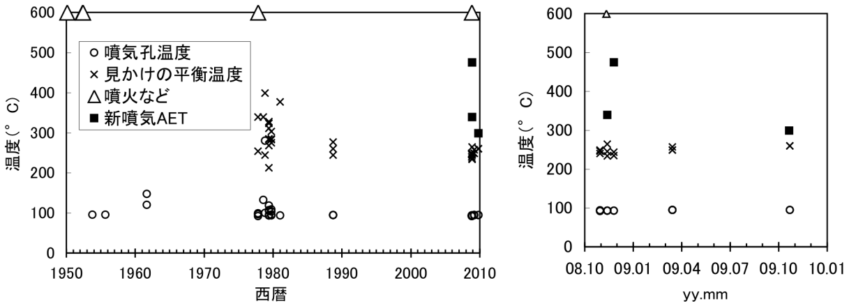
図 1 噴気温度と見かけの平衡温度 (AET: \text{SO}_2+3\text{H}_2=\text{H}_2\text{S}+2\text{H}_2\text{O} )
