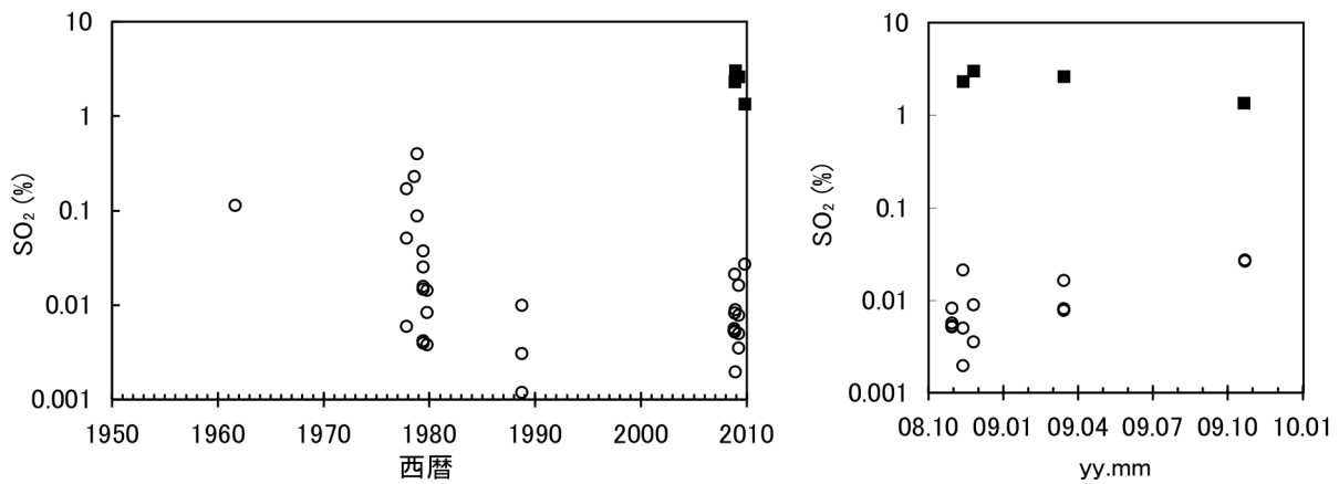
図 2 火山ガス中 \text{SO}_2 濃度 (黒四角は新噴気)
