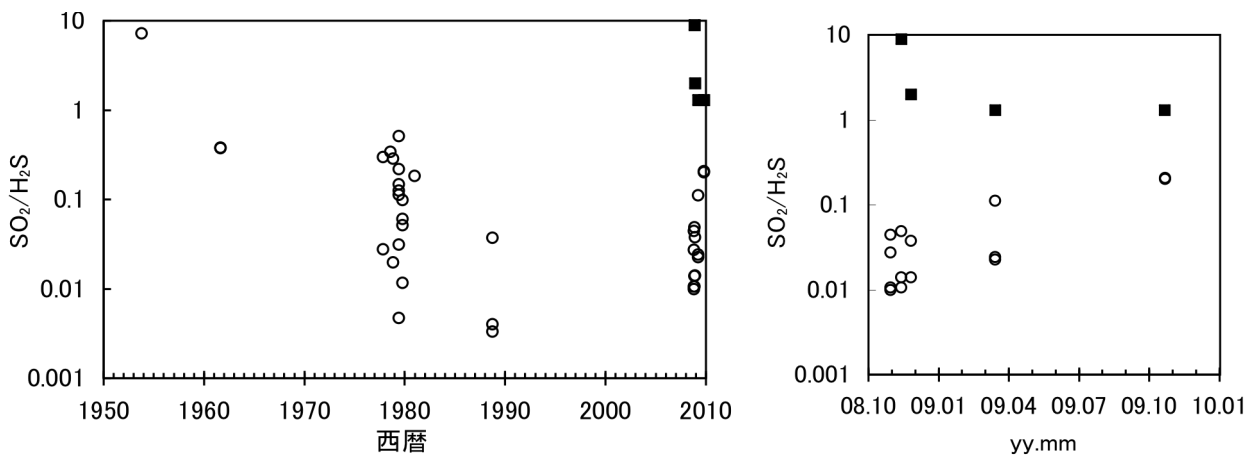
図 3 火山ガス中 \text{SO}_2/\text{H}_2\text{S} 比 (黒四角は新噴気)
