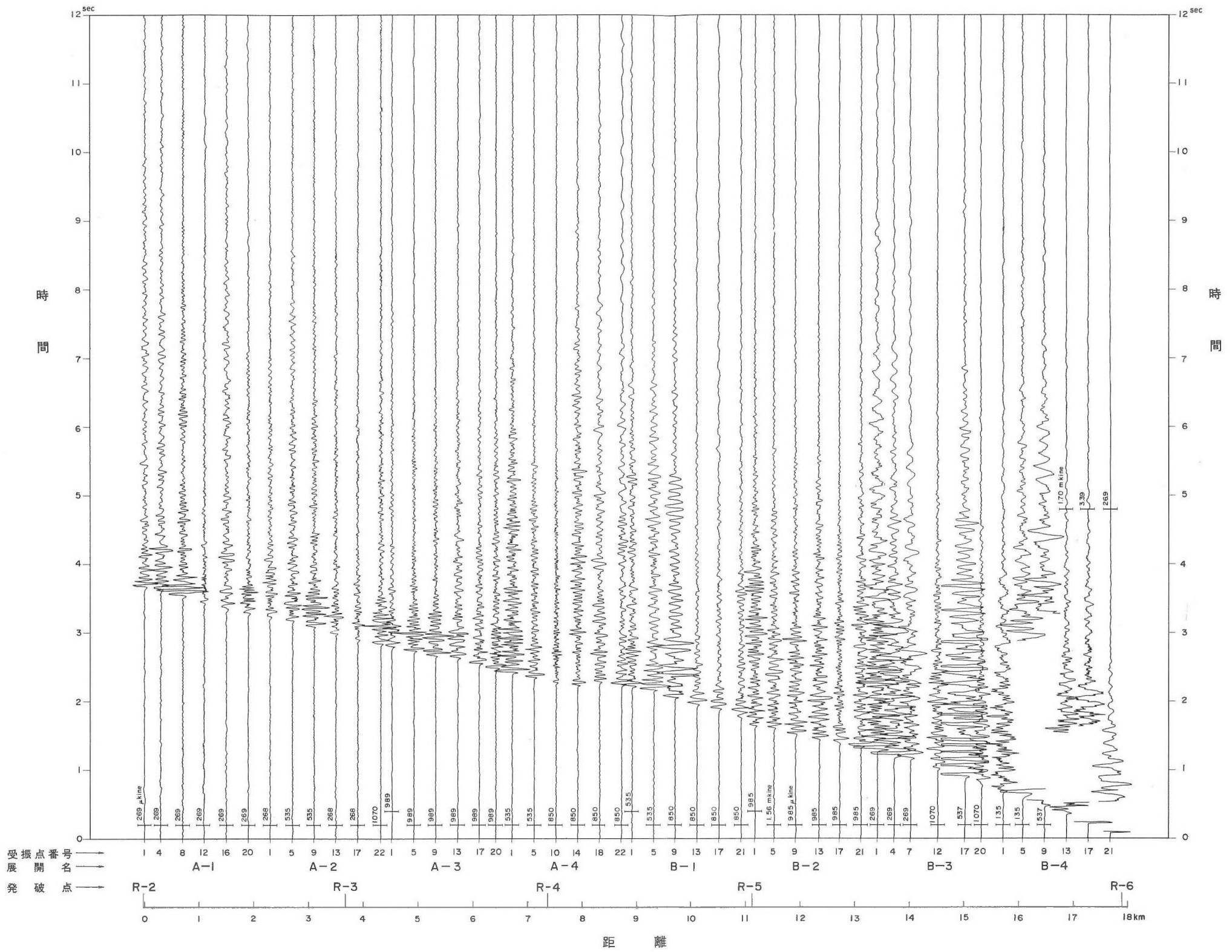
第2(c)図 ショットポイント6のベストアップ図 (新エネルギー総合開発機構, 1982a). Fig. 2(c) Record section (shot 6).
