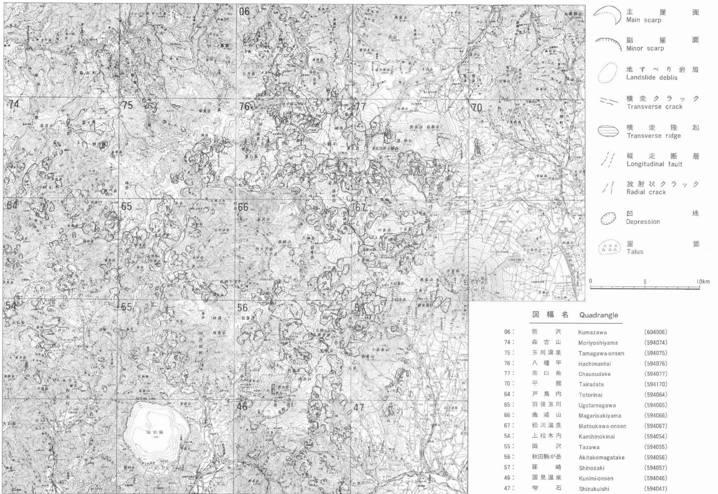
第4-1図 仙岩地熱地域及びその周辺の地すべり地形の分布—その1, 全域。 Fig. 4-1 Distribution of landslide landforms in Sengan geothermal area and its environs—no. 1 whole area.
