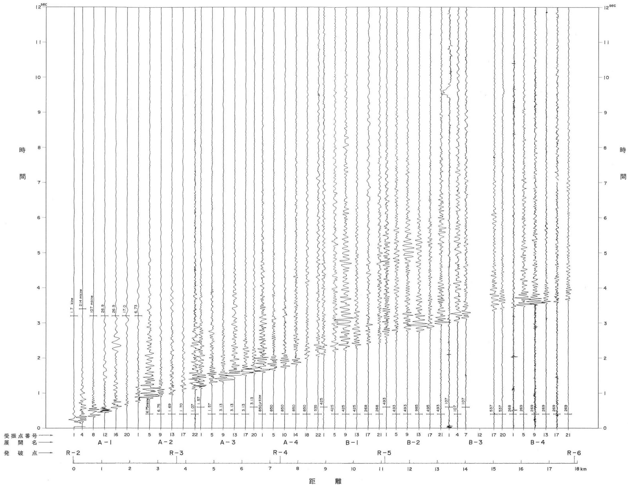
第2(a)図 ショットポイント2のペーストアップ図 (新エネルギー総合開発機構, 1982a). Fig. 2(a) Record section (shot 2).
