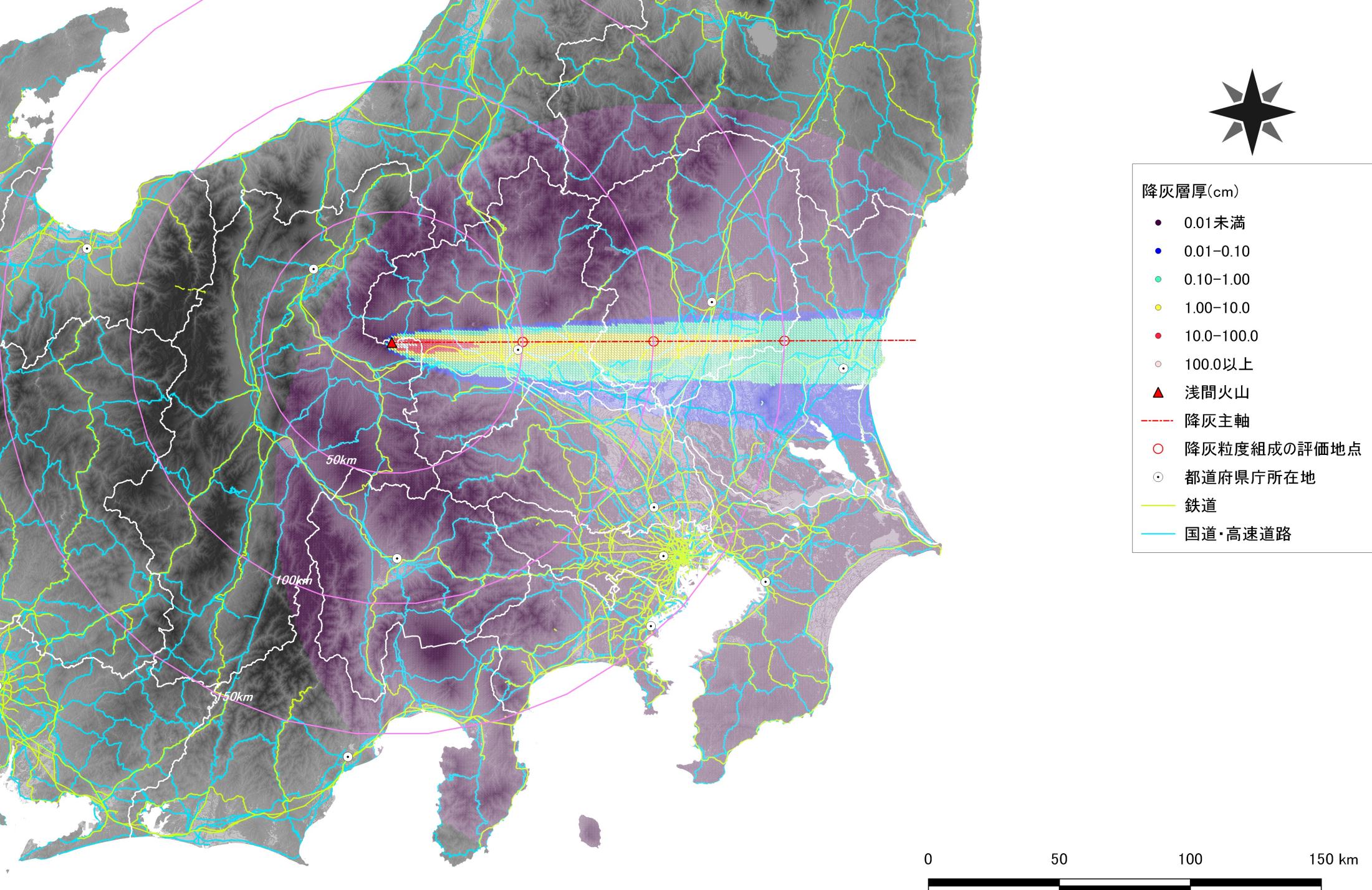
天明噴火規模の月ごとの出力による4月の降灰層厚の分布
