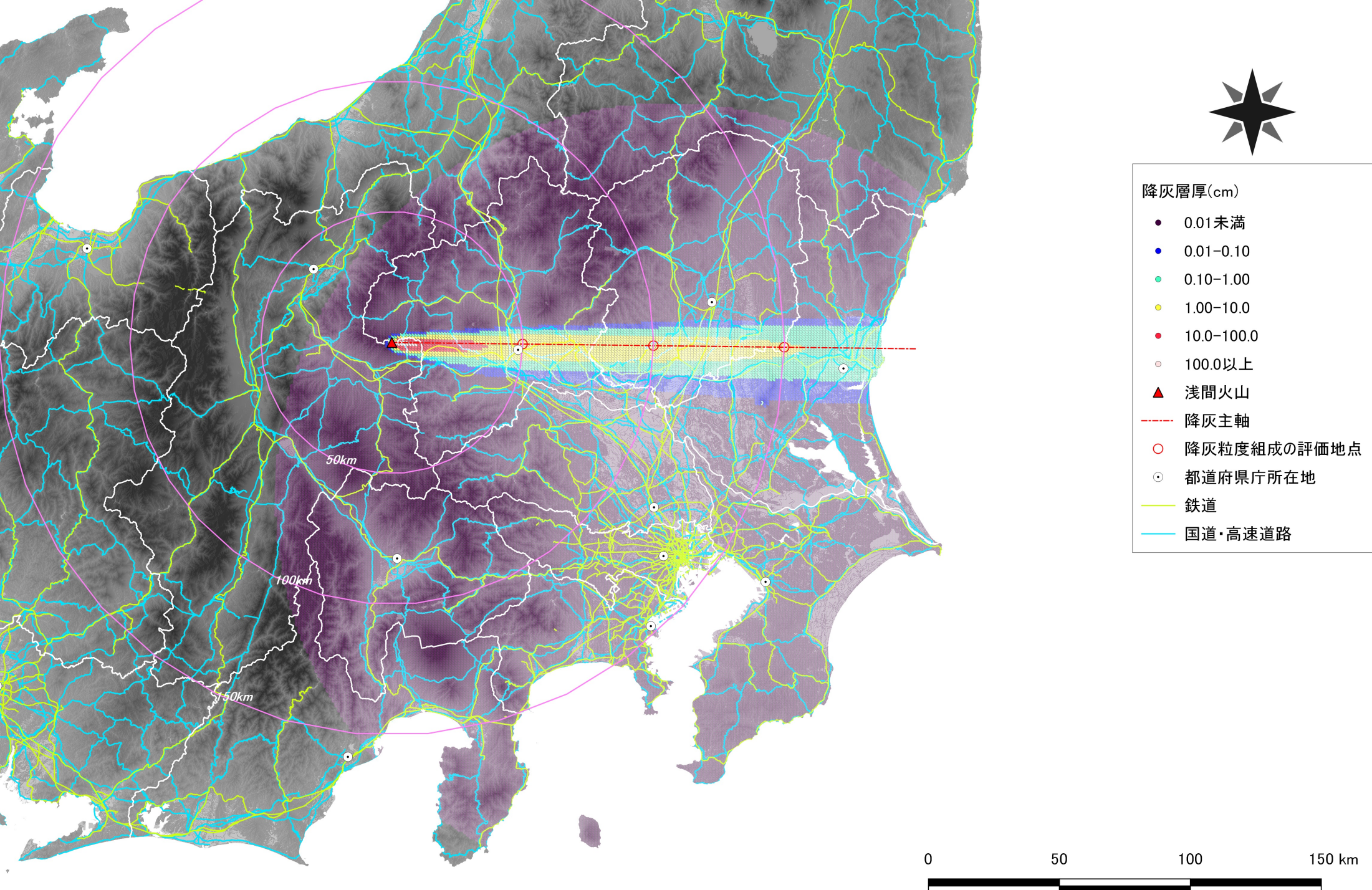
天明噴火規模の月ごとの出力による2月の降灰層厚の分布
