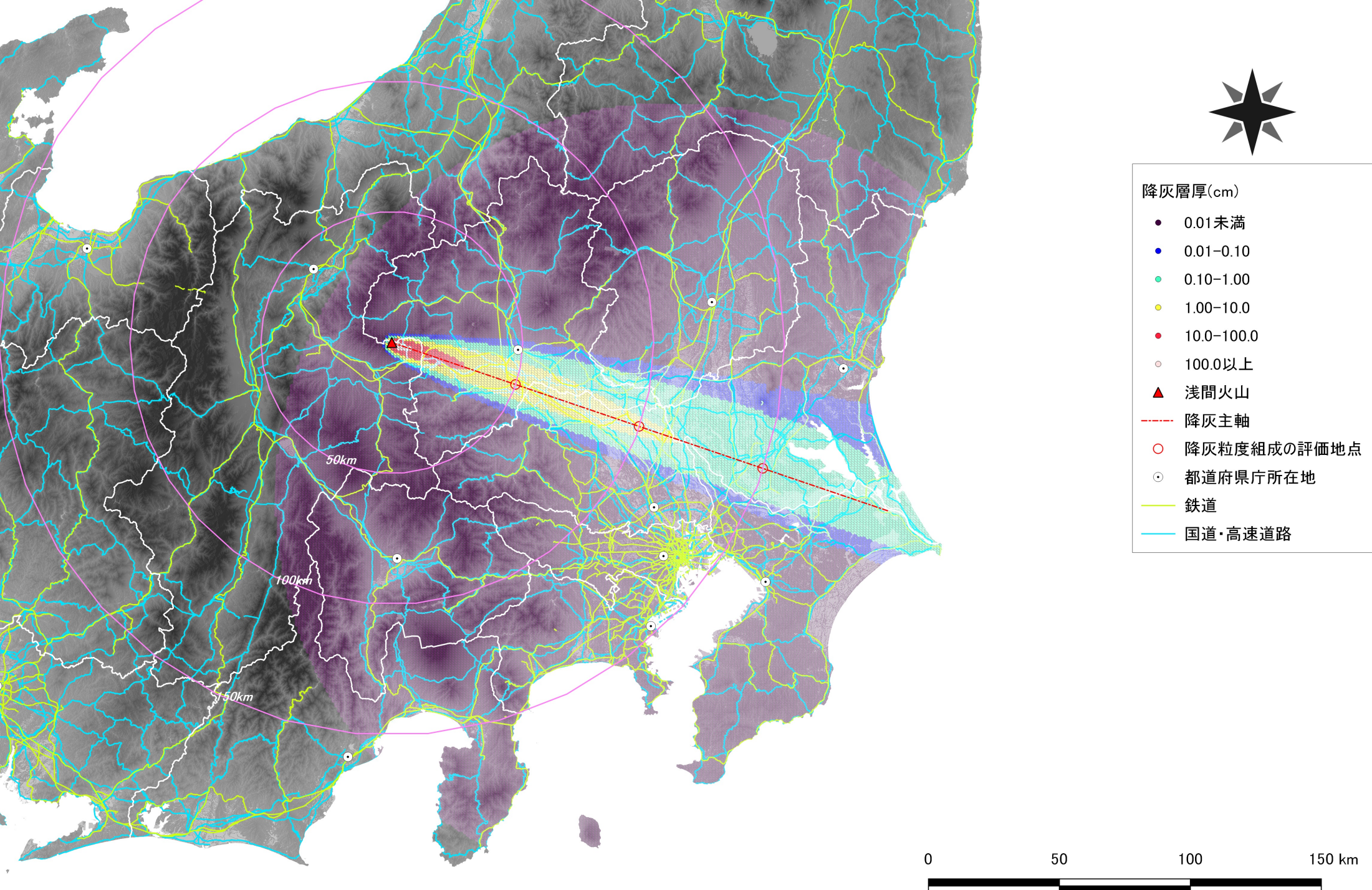
天明噴火規模の月ごとの出力による7月の降灰層厚の分布
