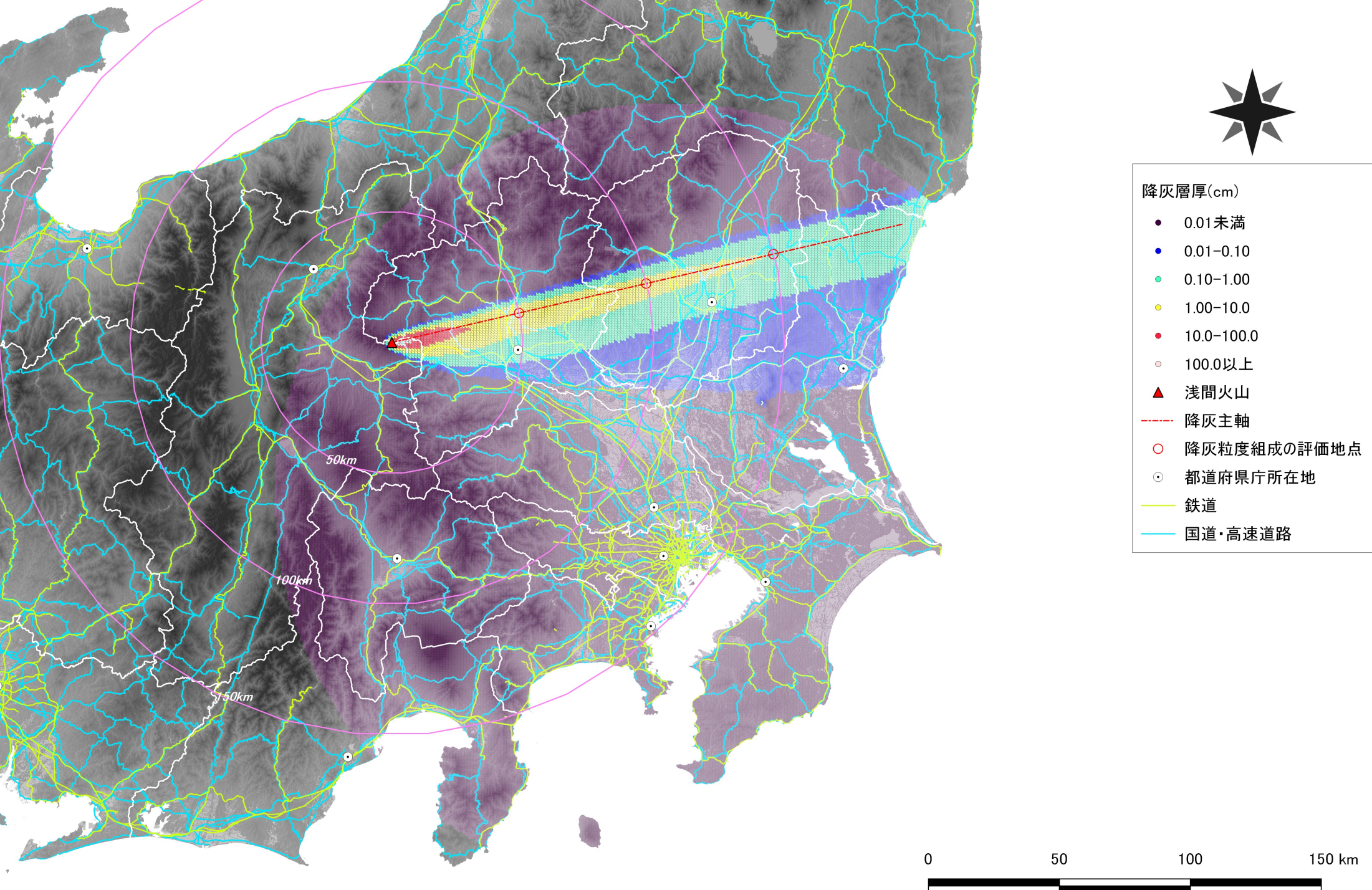
天明噴火規模の月ごとの出力による10月の降灰層厚の分布
