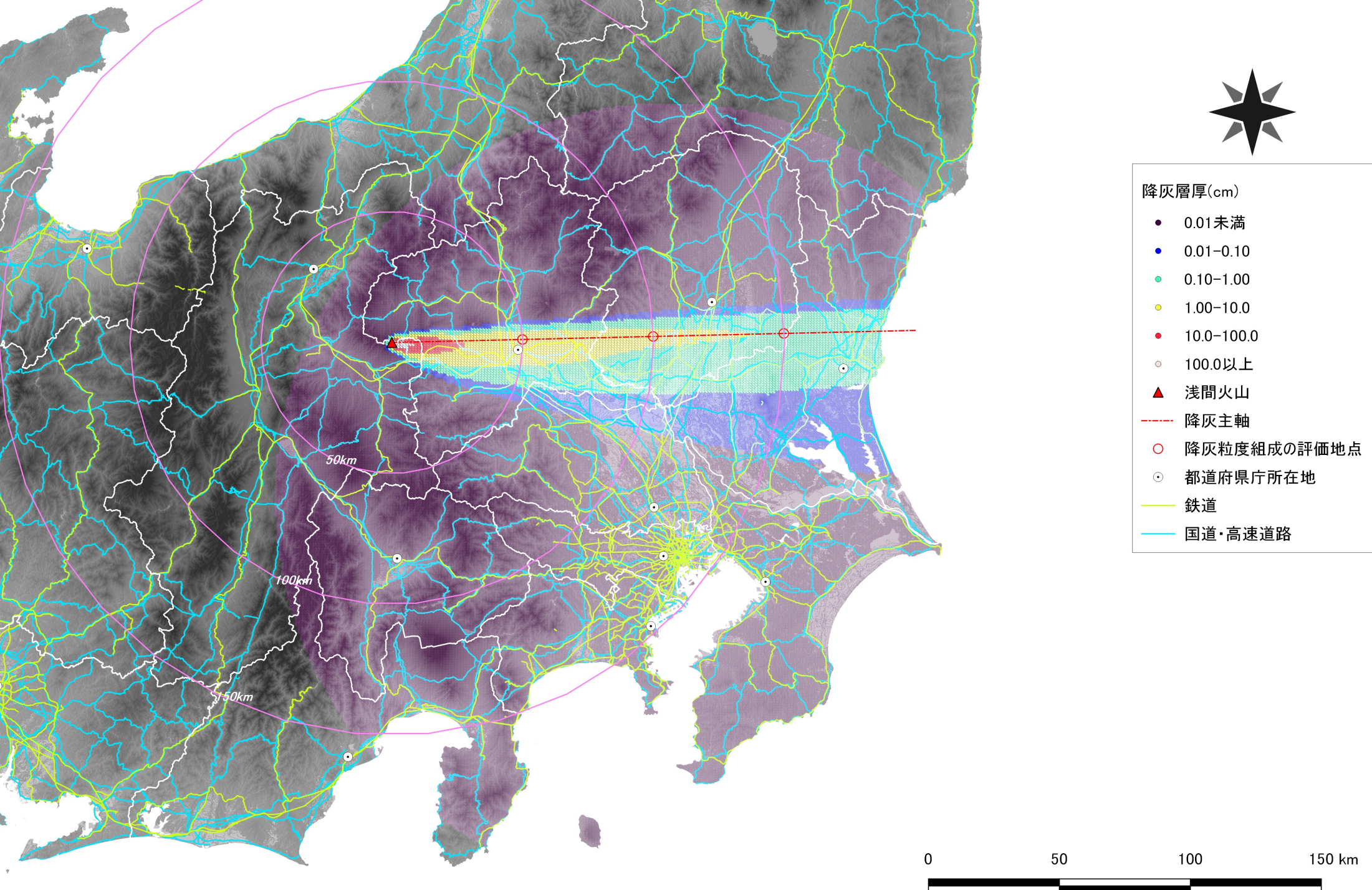
天明噴火規模の月ごとの出力による5月の降灰層厚の分布
