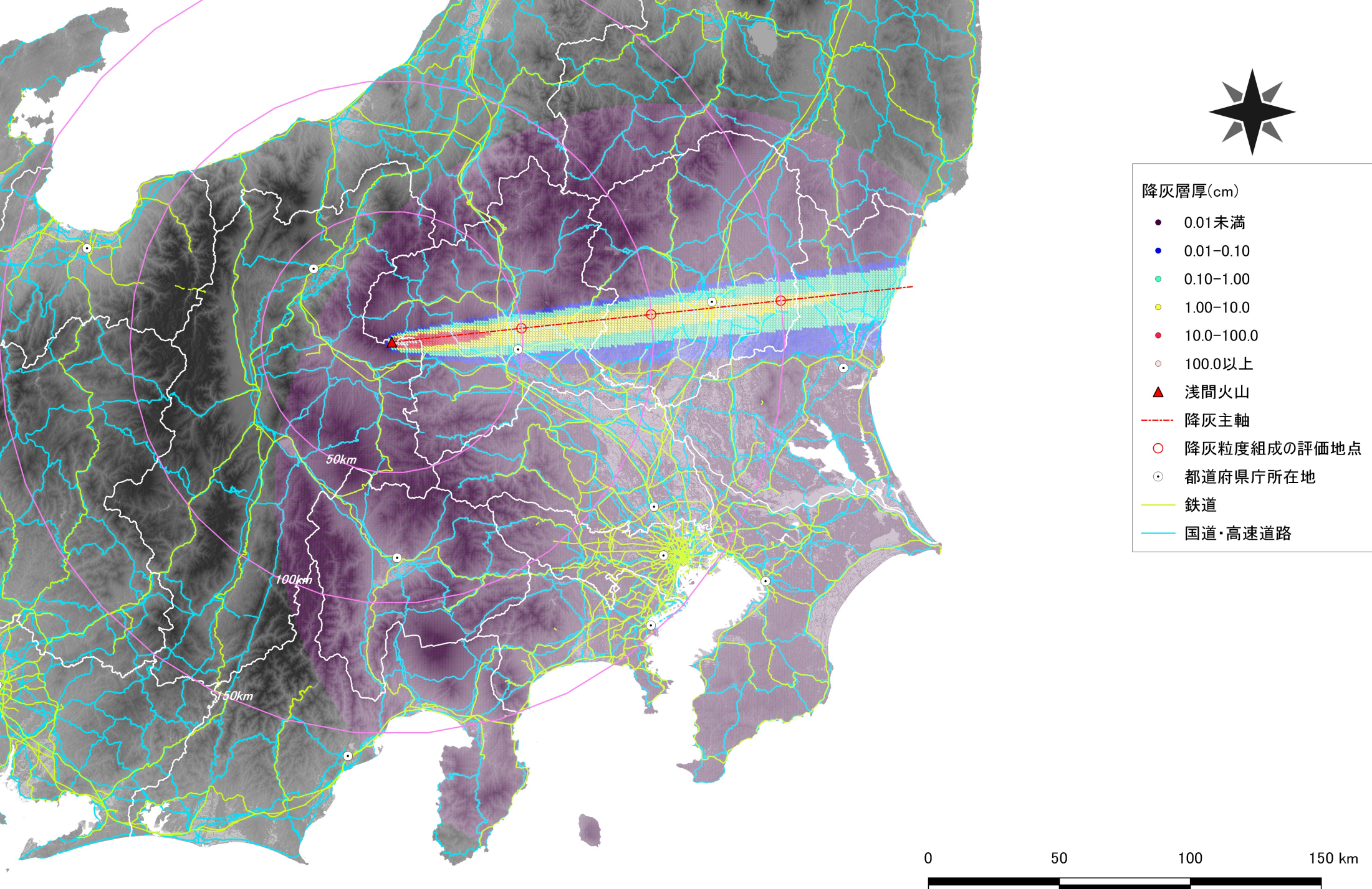
天明噴火規模の月ごとの出力による12月の降灰層厚の分布
