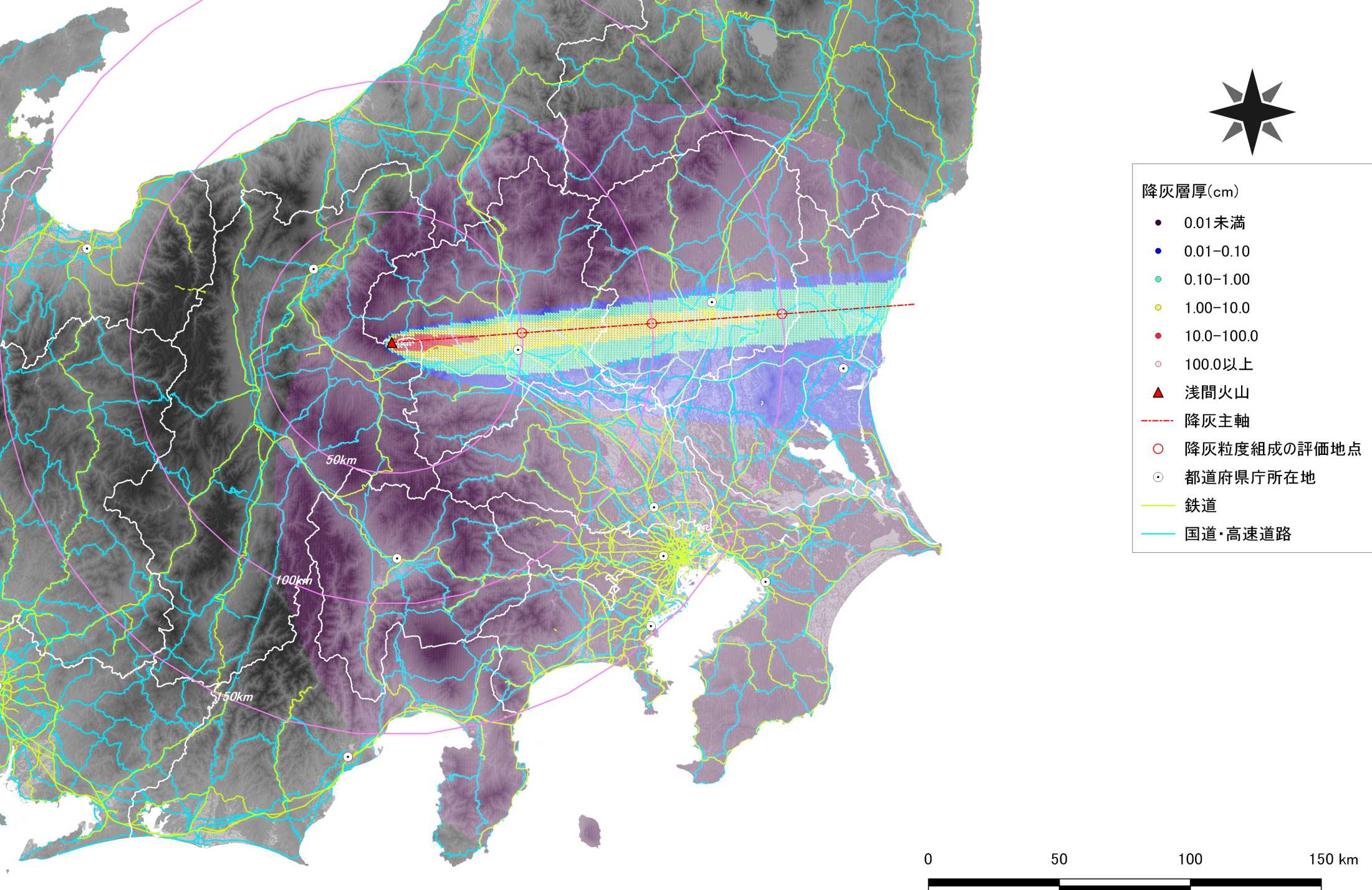
天明噴火規模の月ごとの出力による9月の降灰層厚の分布
