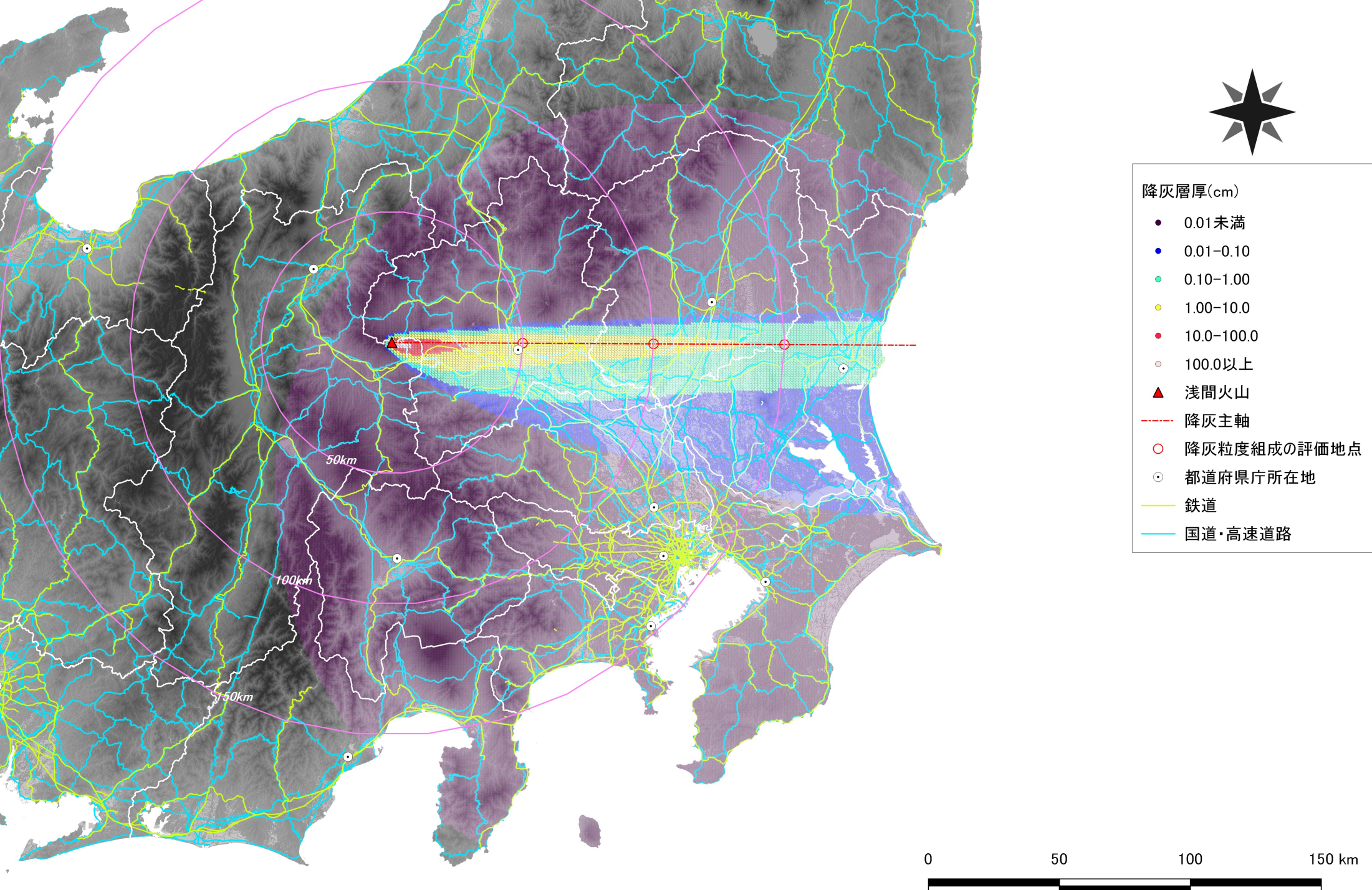
天明噴火規模の月ごとの出力による6月の降灰層厚の分布
