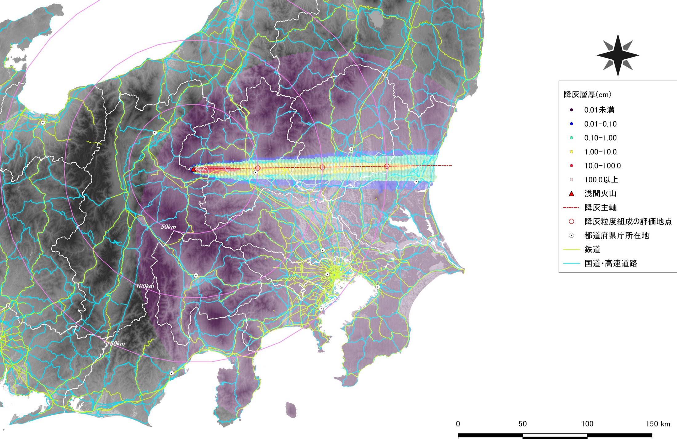
天明噴火規模の月ごとの出力による3月の降灰層厚の分布
