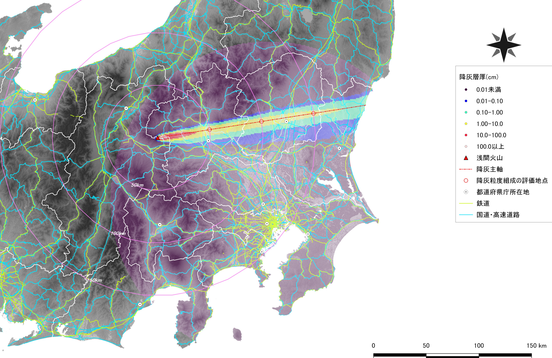
天明噴火規模の月ごとの出力による11月の降灰層厚の分布
