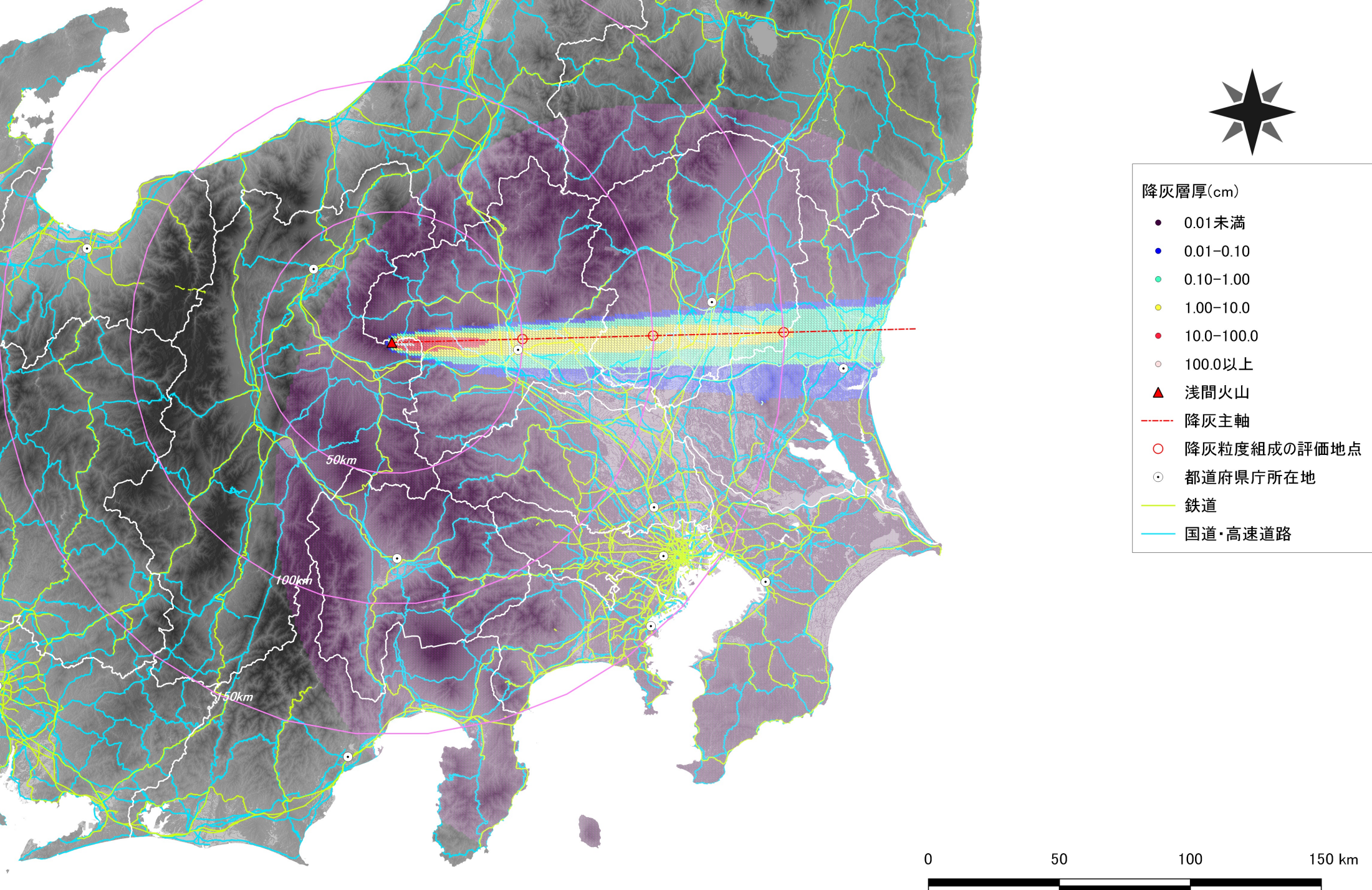
天明噴火規模の月ごとの出力による1月の降灰層厚の分布
