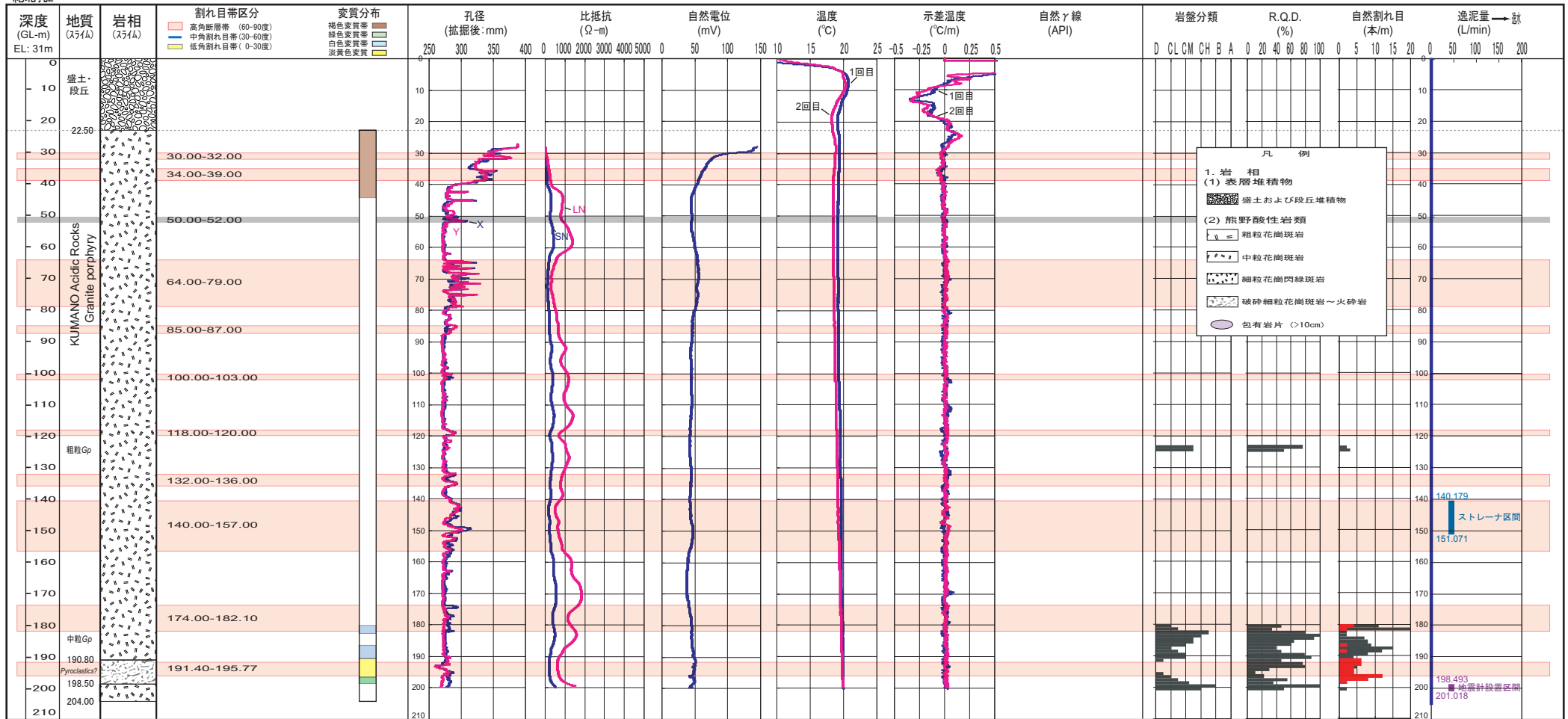
紀北海山観測井-孔2の地質検層柱状図 (0.00-204.00m)
