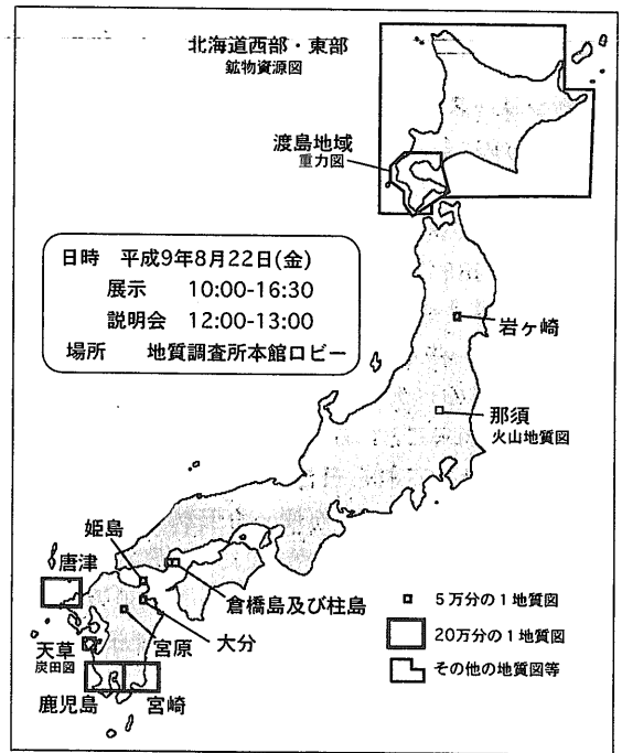
第1図 地質図類の位置図。
