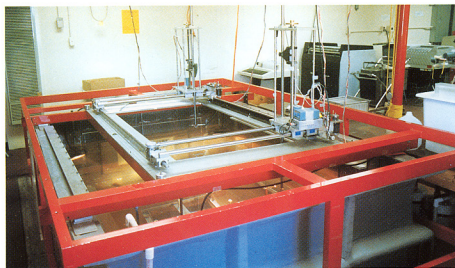
写真1 P波用の実験装置 水槽（音響モデル）
