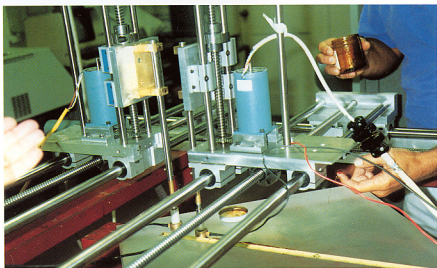
写真1 P波用の実験装置 水槽（音響モデル）
