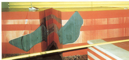
写真2 P波S波両用の実験装置 弾性体モデル用（S波用）
