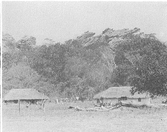
第3図 ムブレの背後に迫る先カンブリア時代の結晶片岩の崖と民家
