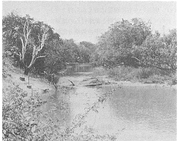
第11図 バミンギの放射能異常地付近 放射能異常は左側の立木の向う側で発見された この川では長さ 60cm ぐらいのスズキに似た魚が簡単に釣れる
