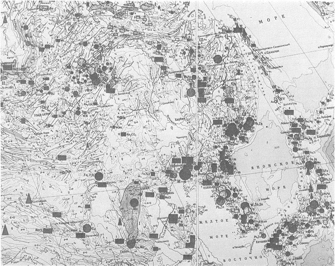
「世界大陸鉱物資源分布図 (Карта полезных ископаемых континентов мира)」 1972
