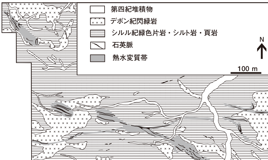
第18図 オロンオボート地域地質図 (Jargalsaihan, 1996)
