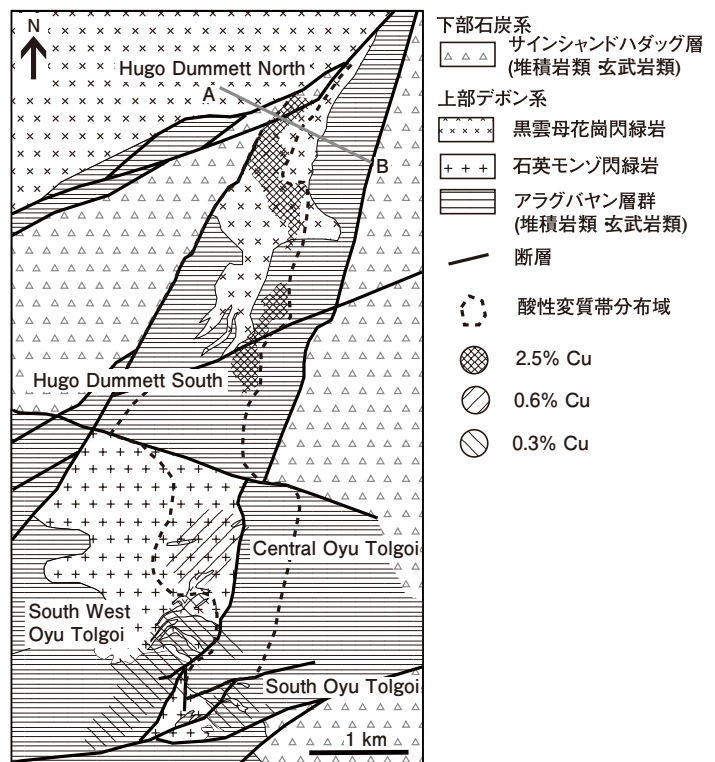
第13図 オユトルゴイ地域地質図. Bat-Erdeneet et al (2005)を簡略化. 潜頭性の銅鉱化部は地表地質図に投影.
