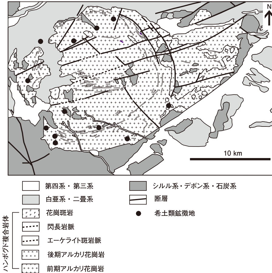
第22図 ハンボグド地域の地質図 (Burenhun et al, 1991).
