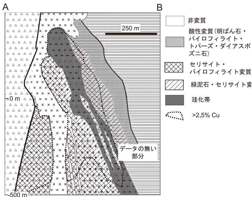
第14図 オユトルゴイ Hugo Dummett North 鉱体断面図. Bat-Erdene et al (2005)を簡略化. 断面位置および岩石種は第13図参照.
