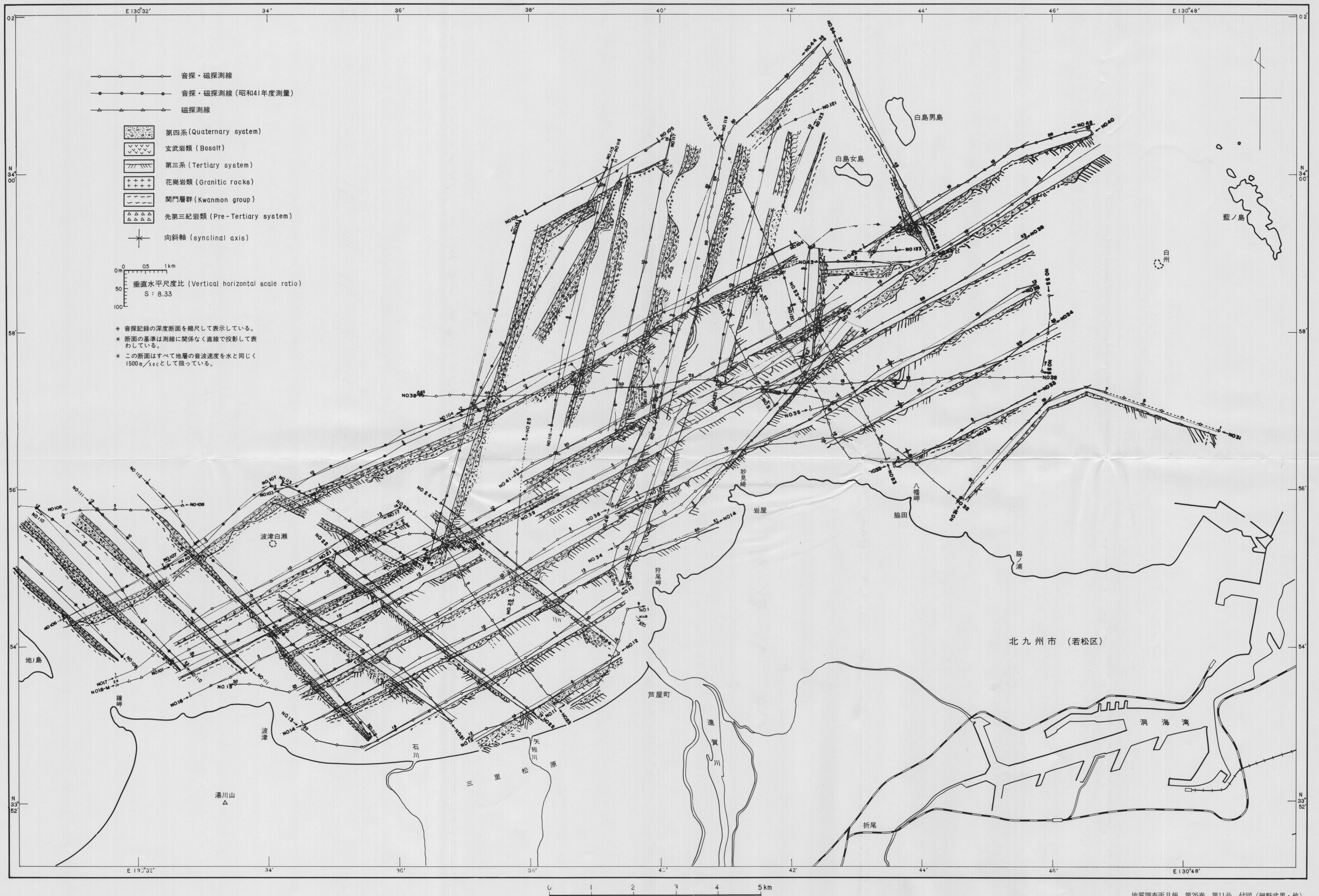
第4図 北九州市西方海域音波探査解析断面図 Fig. 4 Interpreted Cross Sections of Sparker's Reflection Profile off Kitakyushu City
