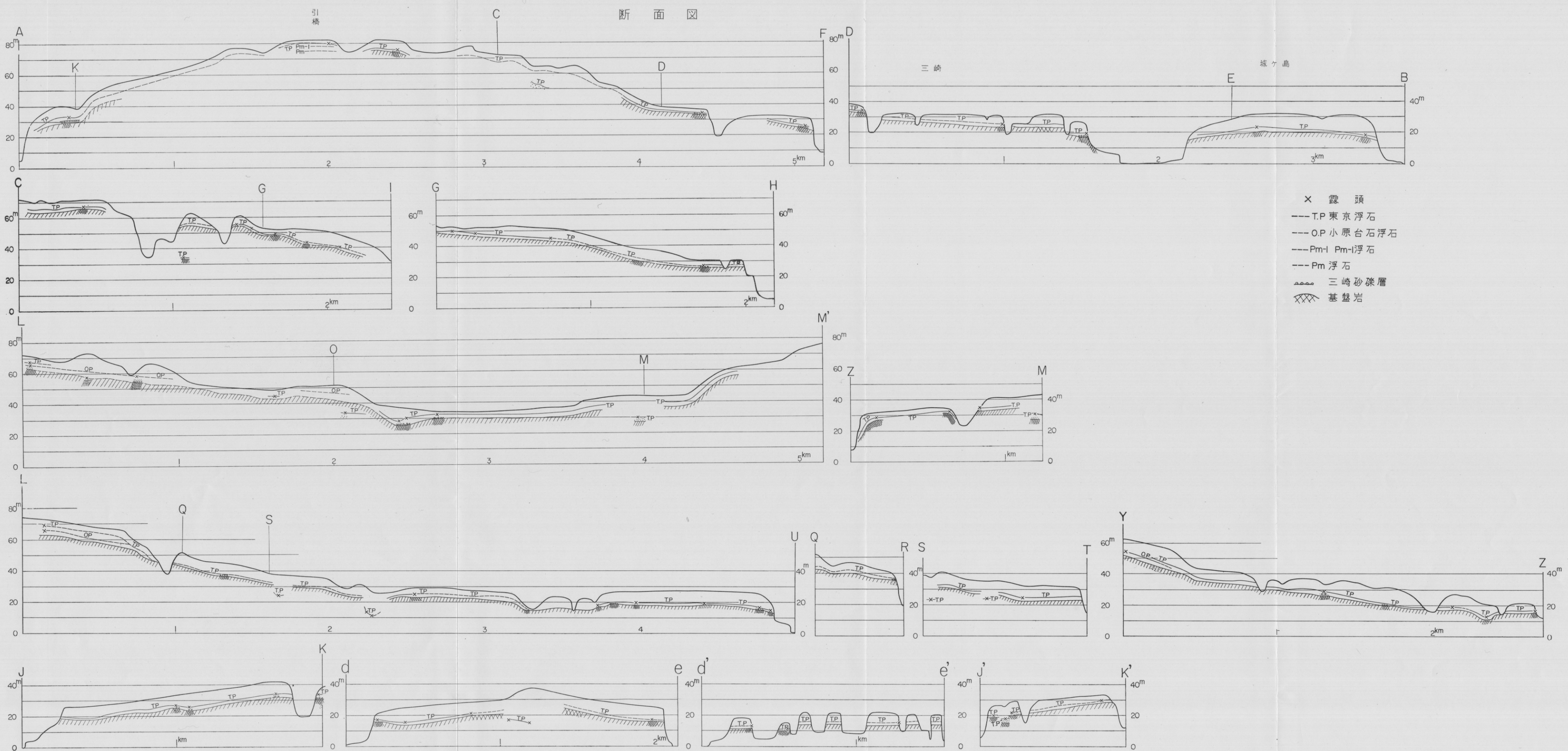
第8図 三崎面の断面図
