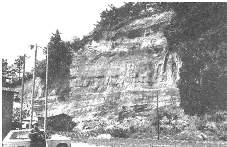
図版 9 浜名郡庄内村平松における佐浜泥層とその下部に発達する砂礫層およびその上部をおおう三方ヶ原礫層（地点11a）
