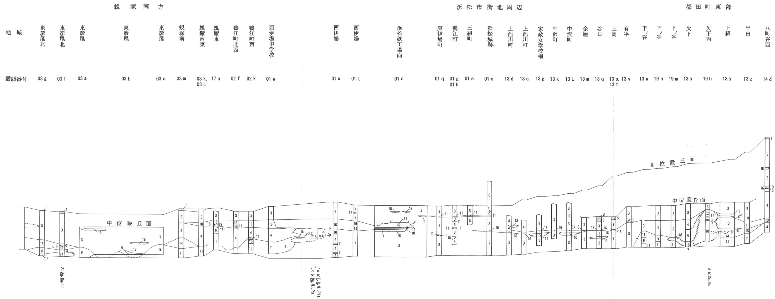
第 12 図 三方が原地周辺第四系柱状対比図 1
