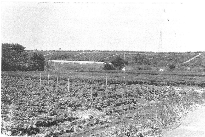
図版 4 三方ヶ原東縁部における中位段丘面上よりみた高位段丘面 (浜松市東三方町北藪付近)
