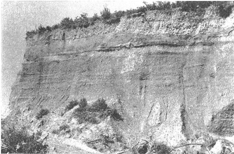
図版 12 浜松市東三方町内野西の崖に見られる三方ヶ原礫層(上部)と 浜松累層曳馬砂礫層(上部に泥層約1.8mを挟む)
