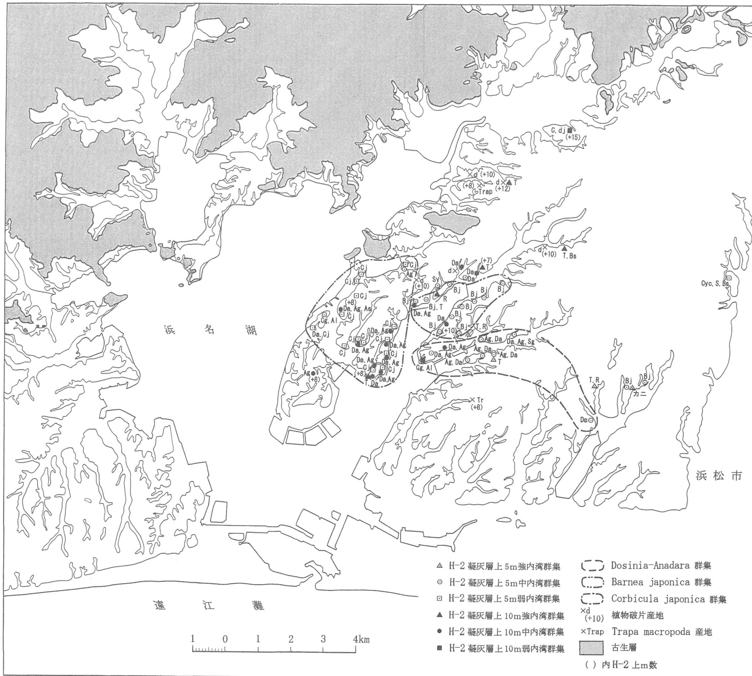
第 16 図 浜松累層産化石群集の分布 H-2凝灰岩層上5mおよび10m層準の化石群集
