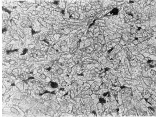
第16図 中粒輝緑岩の顕微鏡写真 ×50
