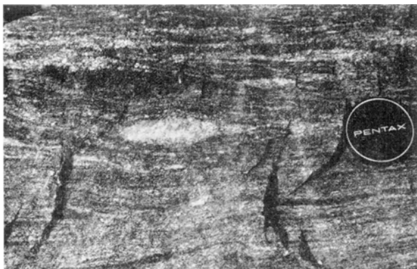
第9図 縞状黒雲母片麻岩
