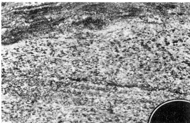
第12図 片麻岩状ミグマタイト
