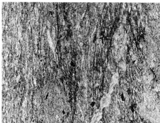
第 7 図 含堇青石ホルンヘルスの顕微鏡写真 × 50
