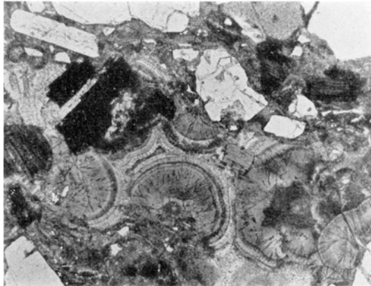
第5図 十勝熔結凝灰岩の顕微鏡写真 ×50
