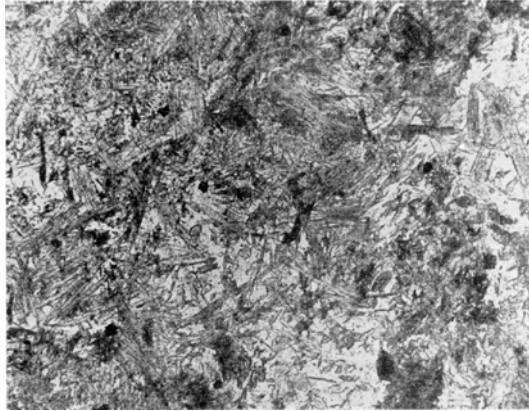
第 8 図 緑色岩類の顕微鏡写真 × 50
