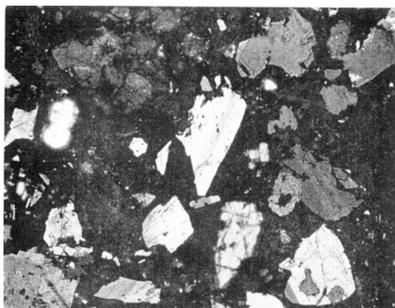
第 7 図 第 1 熔結凝灰岩（安山岩質熔結凝灰岩）
