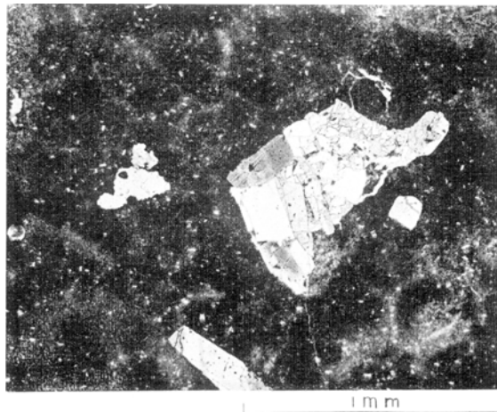
第 10 図 流紋岩脈 (浦島内川)
