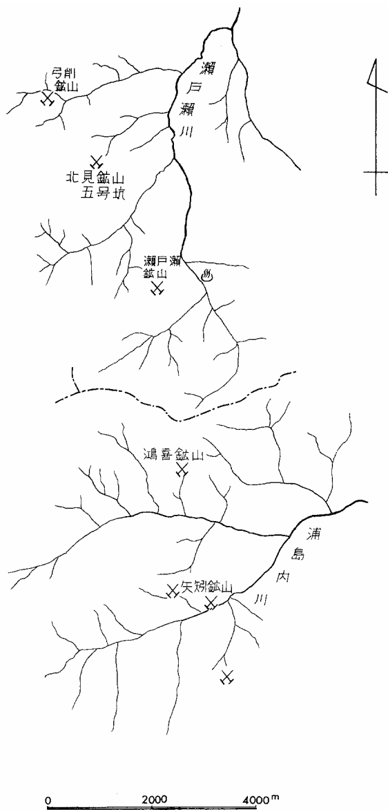
第14図 鉢山分布図
