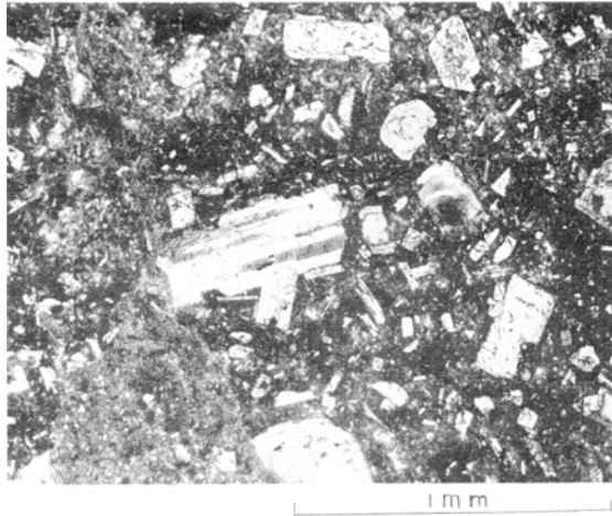
第 13 図 玄武岩質安山岩（武利川）
