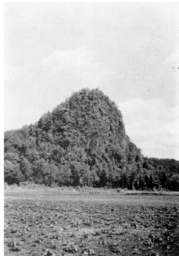
第 5 図 流紋岩
