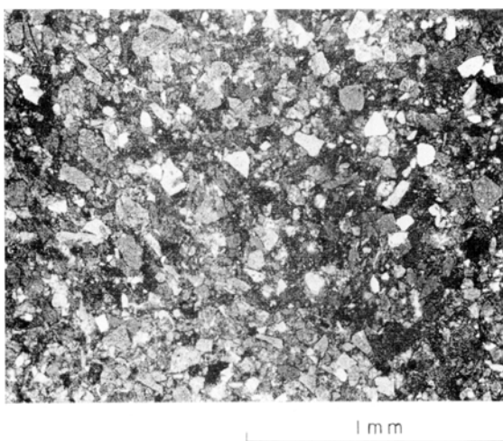
第9図 第3熔結凝灰岩 (大平)
