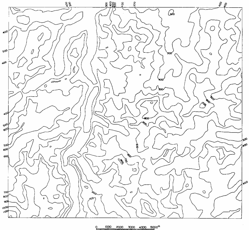
第2図 地形復元図（谷を500mの間隔で埋めて作成した）
